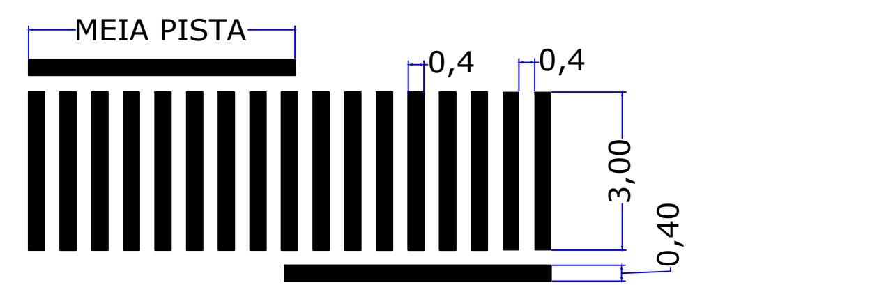
Detalhes da Travessia de pedestres zebraada:
