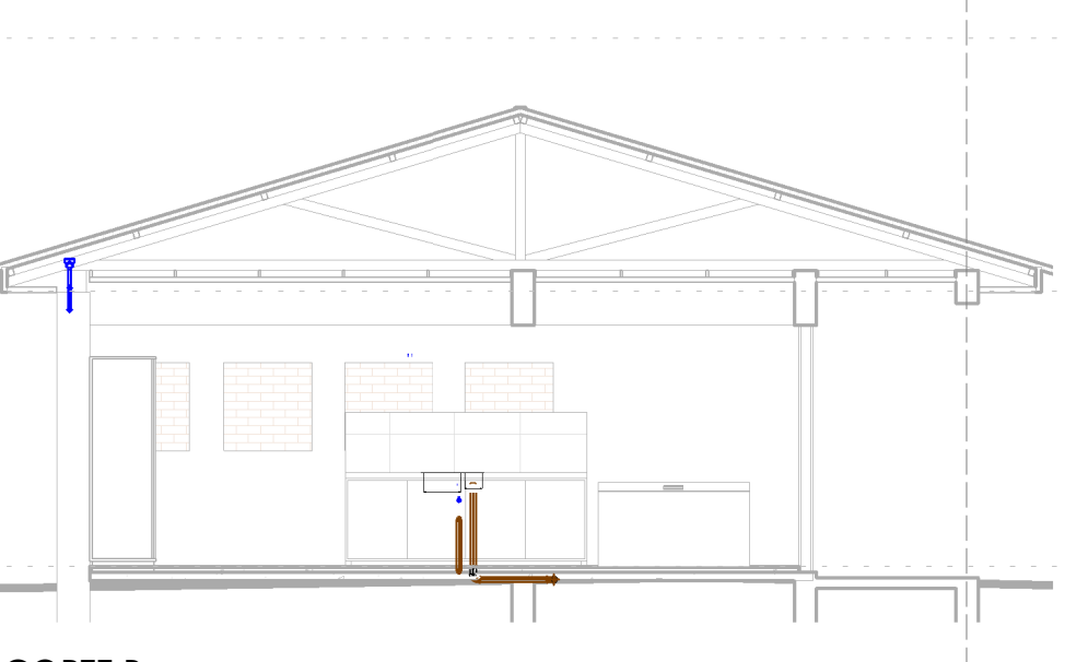
CORTE B ESC:1 : 75
