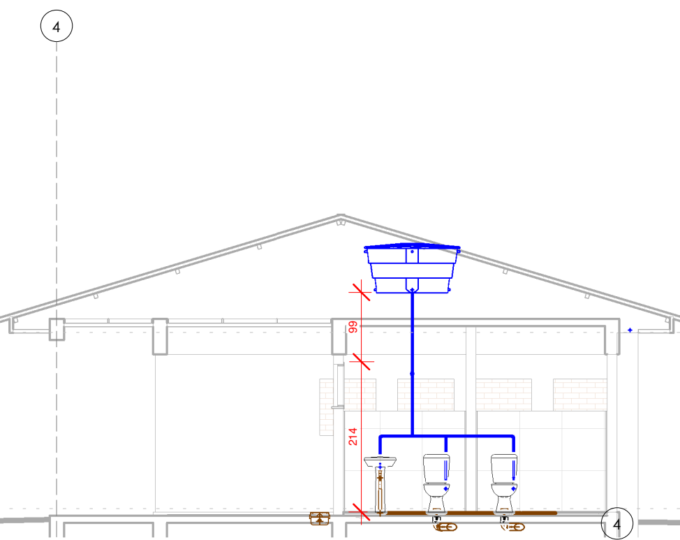
CORTE A ESC:1 : 75
