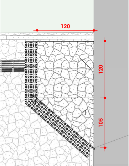
Detalhe Rampa 02 | ESCALA: 1 : 50
