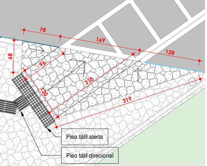
Detalhe Rampa 01 | ESCALA: 1 : 50
