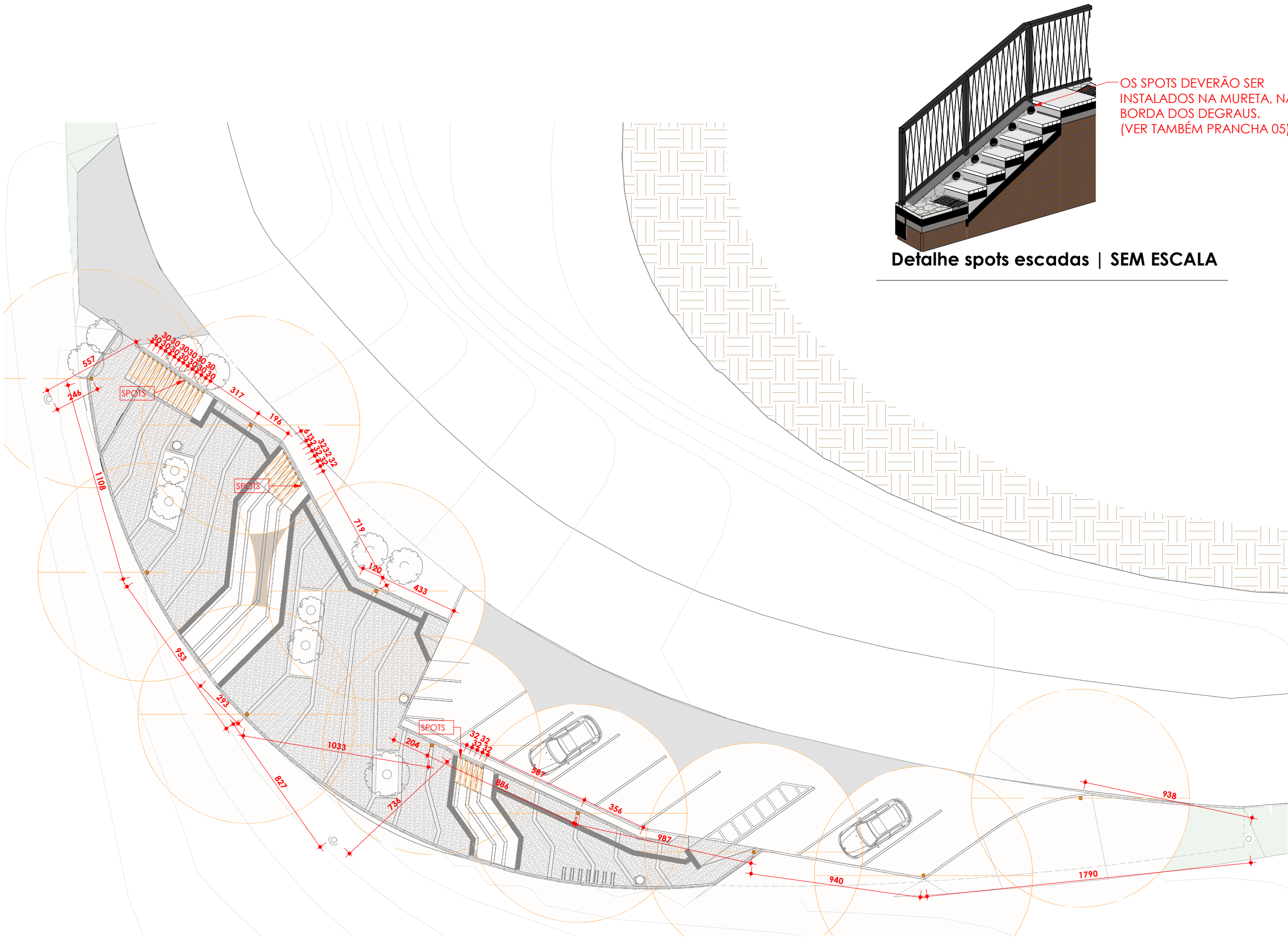
Planta Baixa Iluminação | ESCALA: 1 : 200
