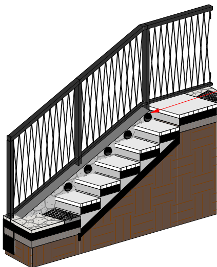
Detalhe spots escadas | SEM ESCALA
