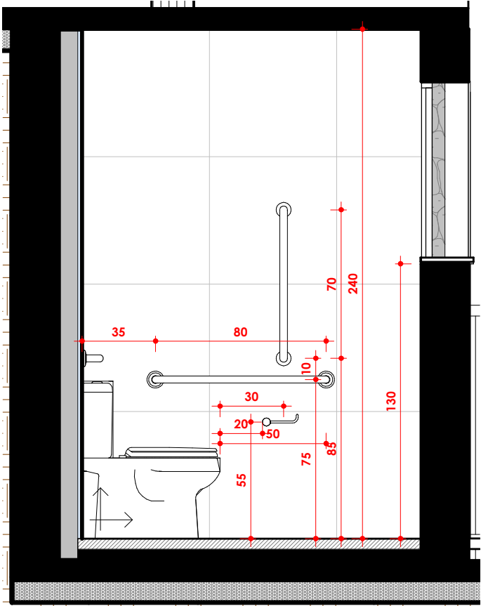
BH 1.2 | ESCALA: 1 : 25
