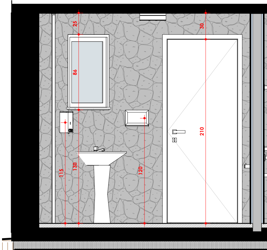
BH 2.3 | ESCALA: 1 : 25
