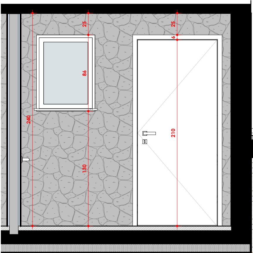
BH 1.3 | ESCALA: 1 : 25
