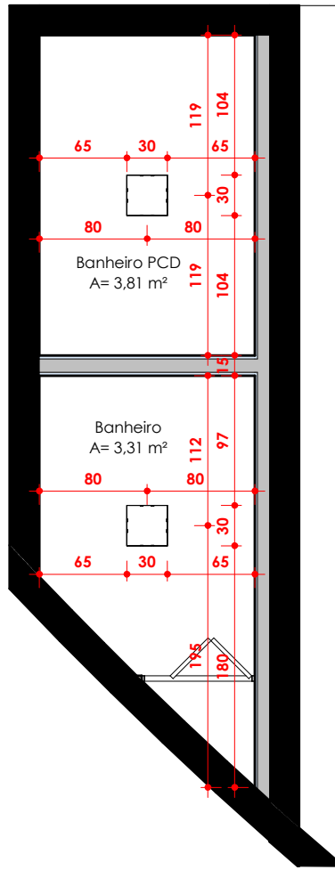
Planta de forro - Banheiros | ESCALA: 1 : 50
