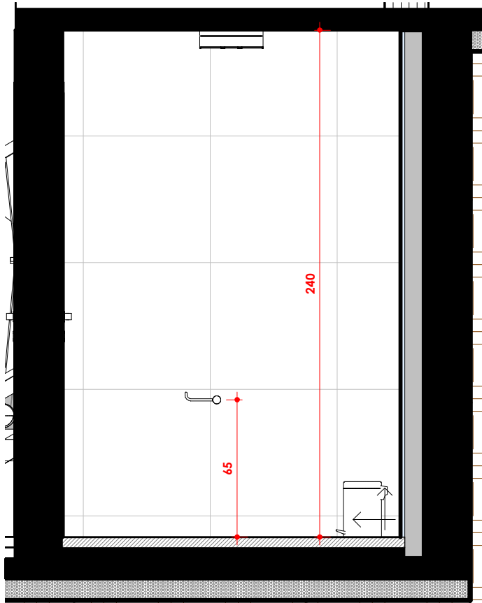
BH 2.4 | ESCALA: 1 : 25
