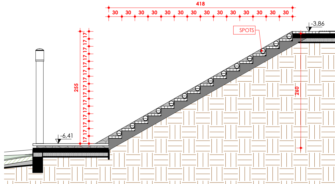
Corte Escada Banheiros | ESCALA: 1 : 50
