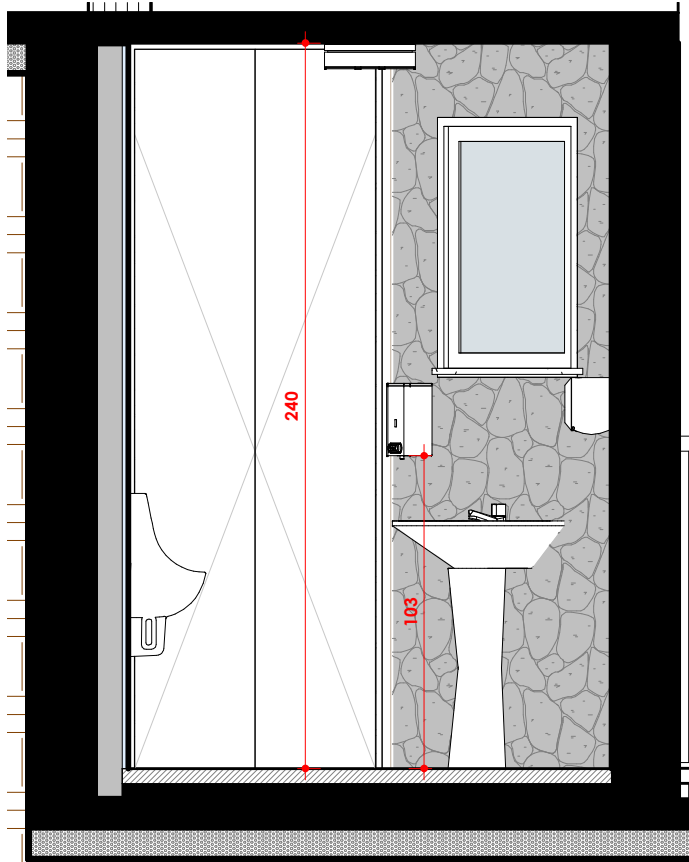
BH 2.2 | ESCALA: 1 : 25
