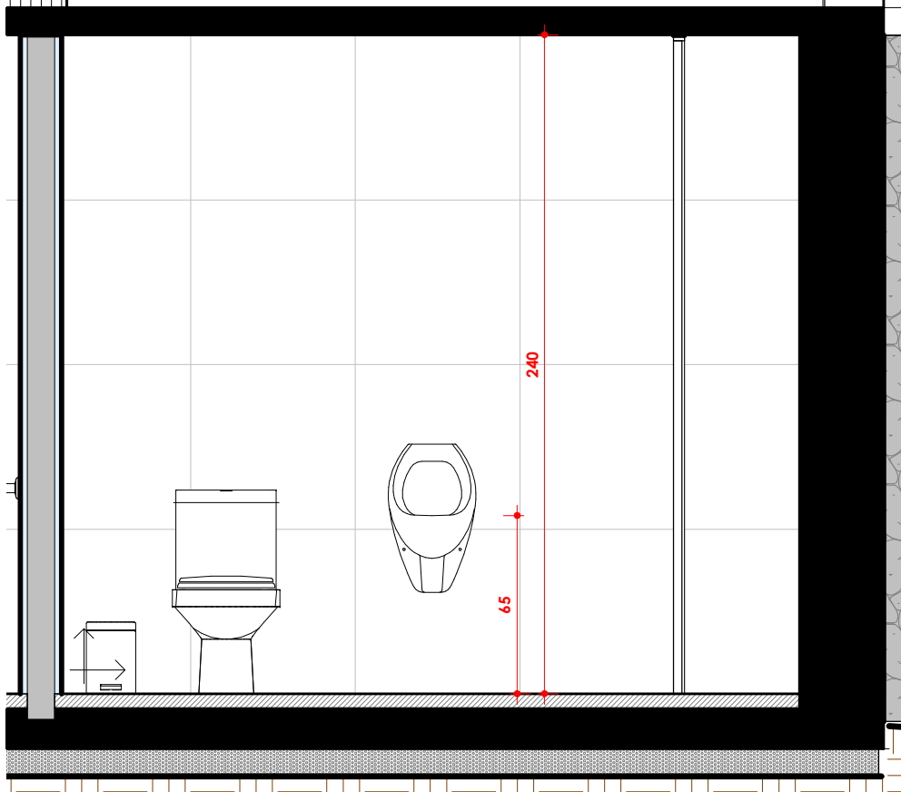
BH 2.1 | ESCALA: 1 : 25
