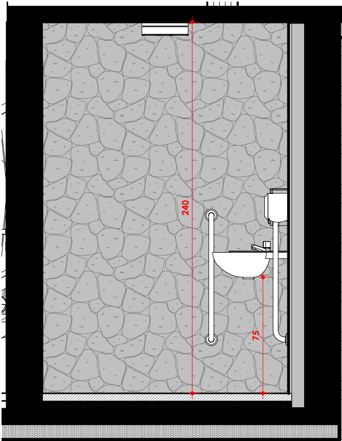
BH 1.4 | ESCALA: 1 : 25
