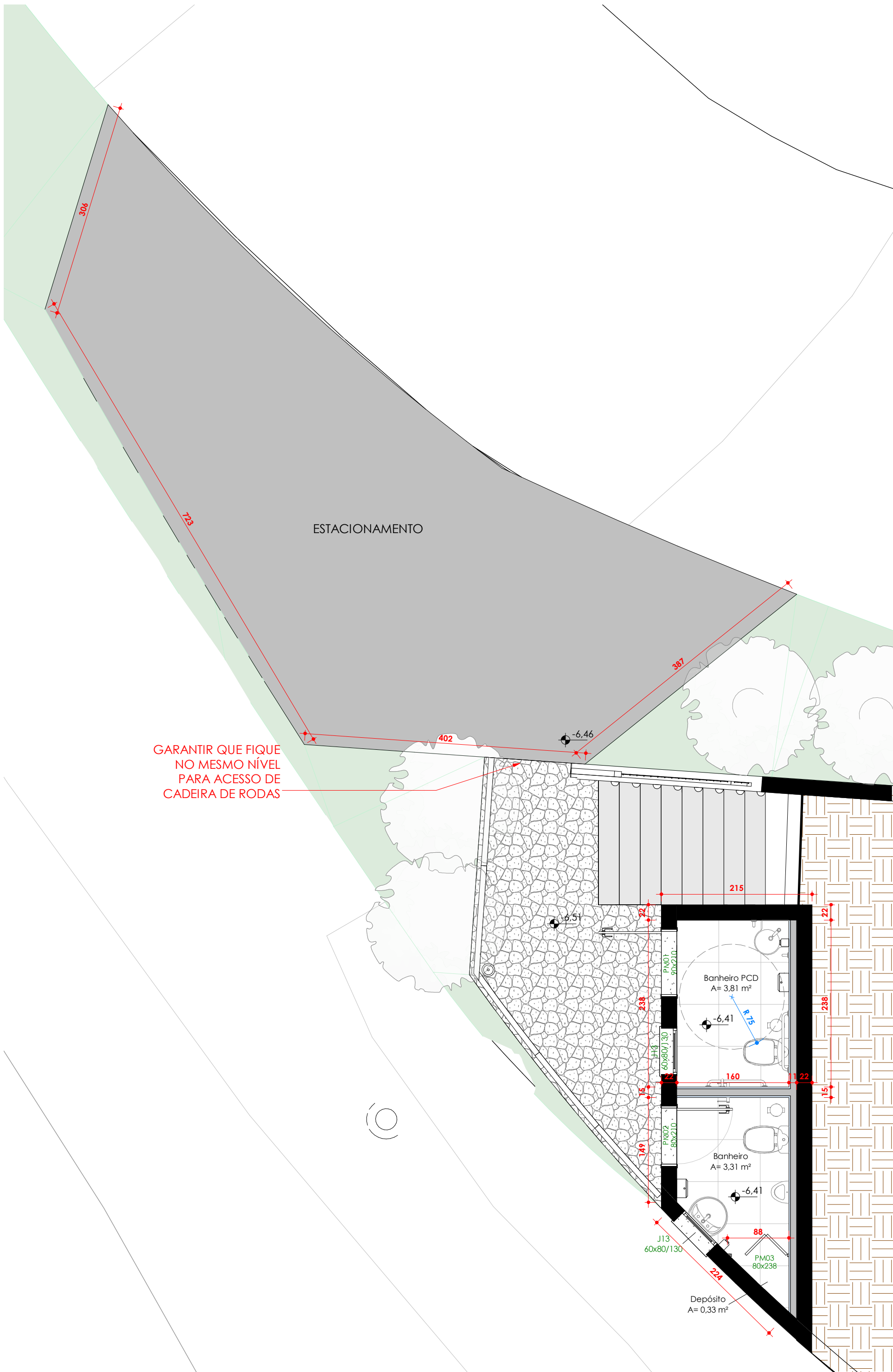
Nível -6_337_Banheiros | ESCALA: 1 : 50
