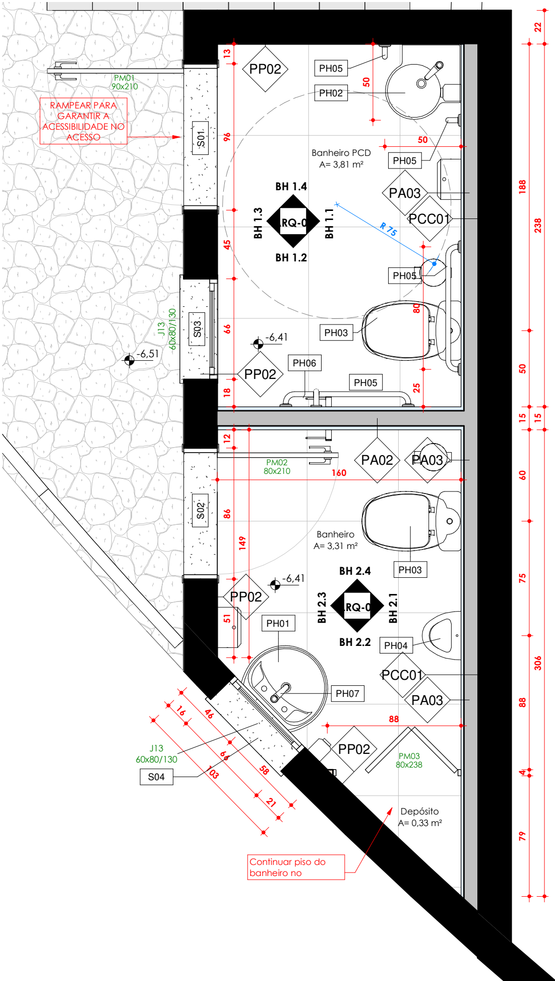
Nível -6_337_Banheiros detalhamento | ESCALA: 1 : 25
