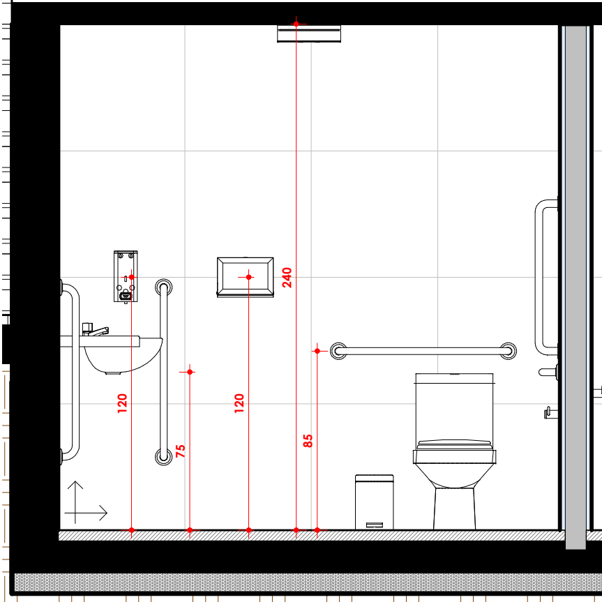
BH 1.1 | ESCALA: 1 : 25
