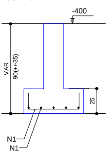
CORTE ESC 1:25
