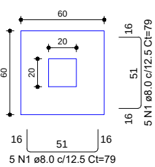
S21 PLANTA ESC 1:25
