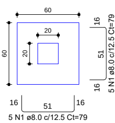
S17 PLANTA ESC 1:25
