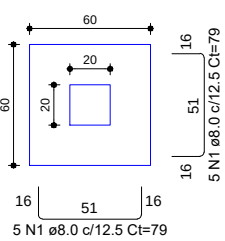
S5=S18=S20 PLANTA ESC 1:25
