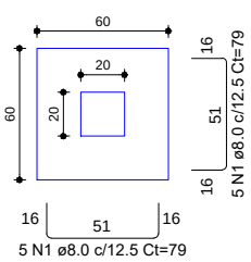
S1=S3=S6=S9=S14 PLANTA ESC 1:25
