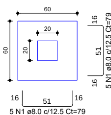
S27 PLANTA ESC 1:25
