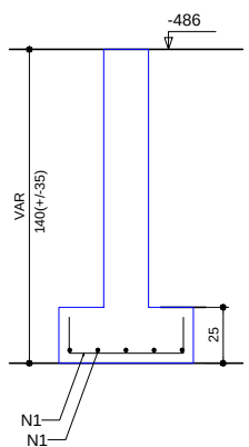
CORTE ESC 1:25
