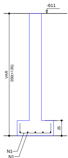
CORTE ESC 1:25
