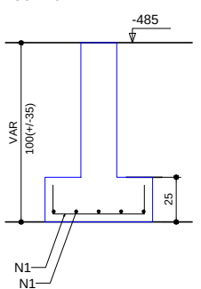
CORTE ESC 1:25
