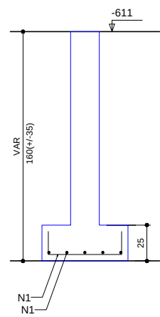
CORTE ESC 1:25
