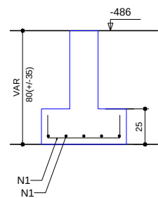
CORTE ESC 1:25
