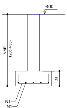
CORTE ESC 1:25
