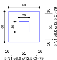
S37 PLANTA ESC 1:25
