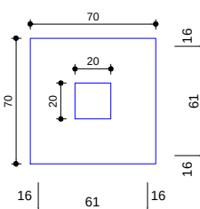
S31 PLANTA ESC 1:25
