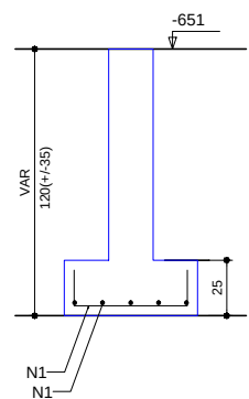
CORTE ESC 1:25
