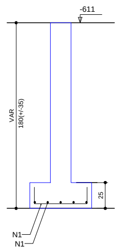
CORTE ESC 1:25
