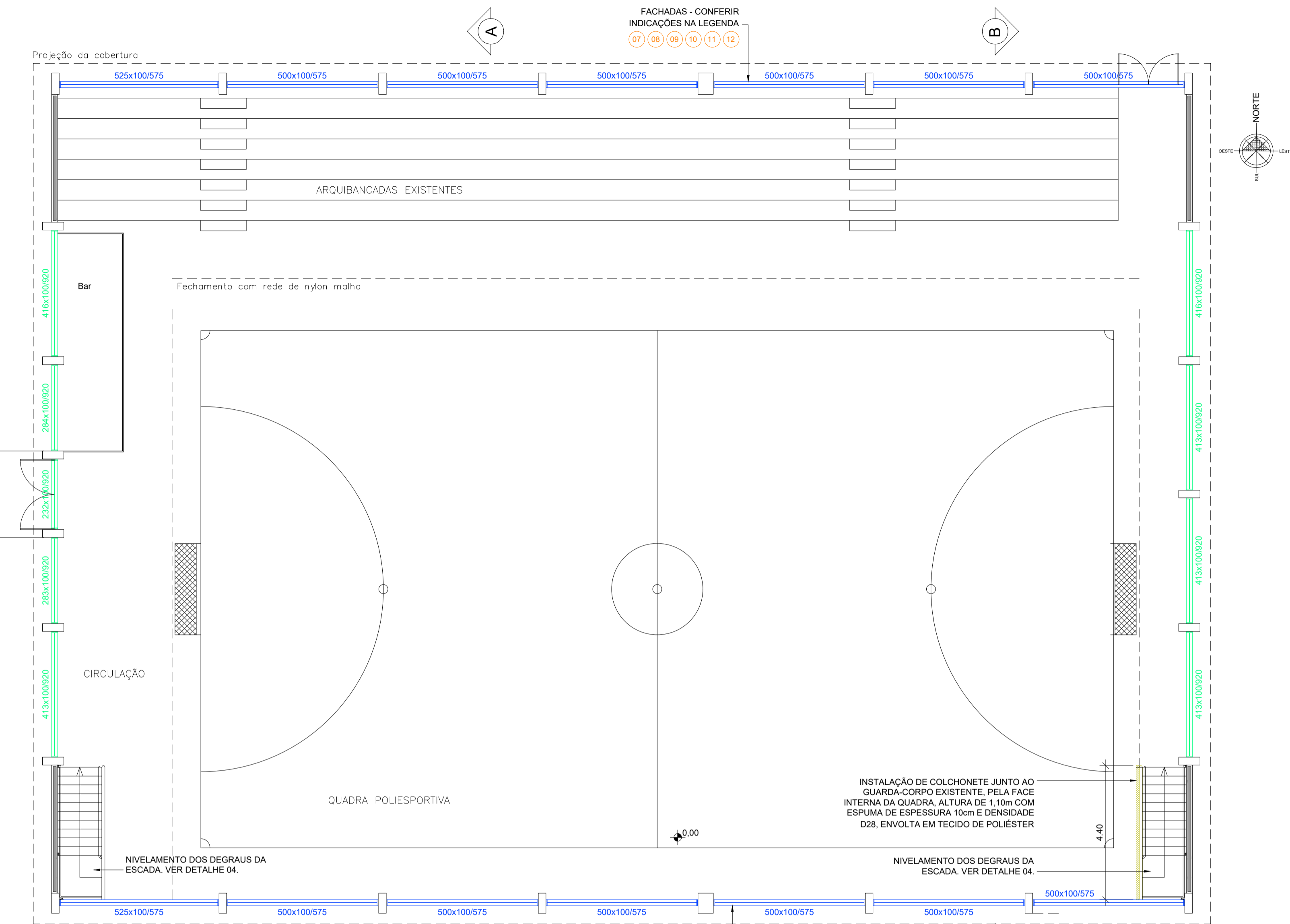
PLANTA BAIXA - REFORMA - CONSTRUIR PAVIMENTO TÉRREO Escala 1:100
