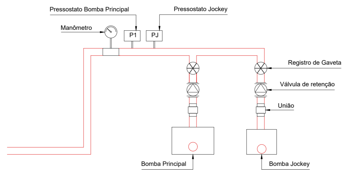
Detalhe Bombas Escala 1:20
