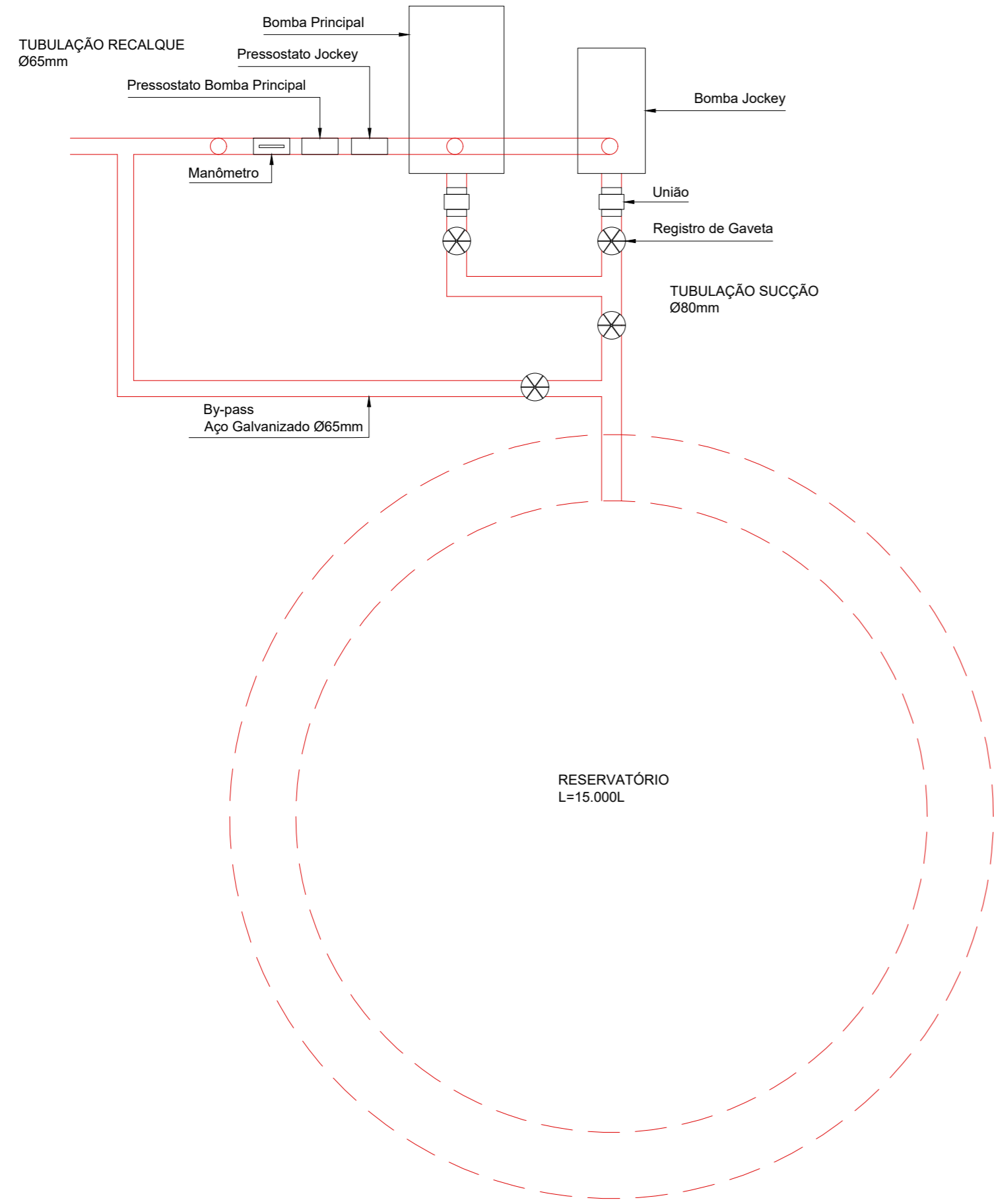
Detalhe 01 – Planta Baixa Escala 1:20
