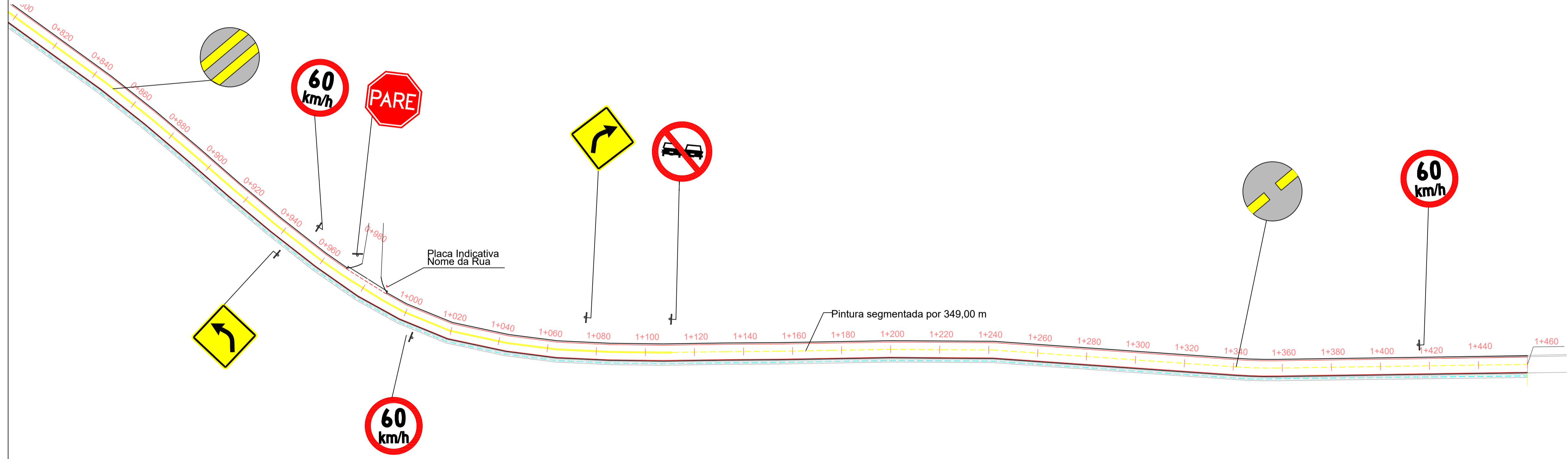
Sinalização Trecho 1 - 0+000 a 0+820 Escala 1/1000
