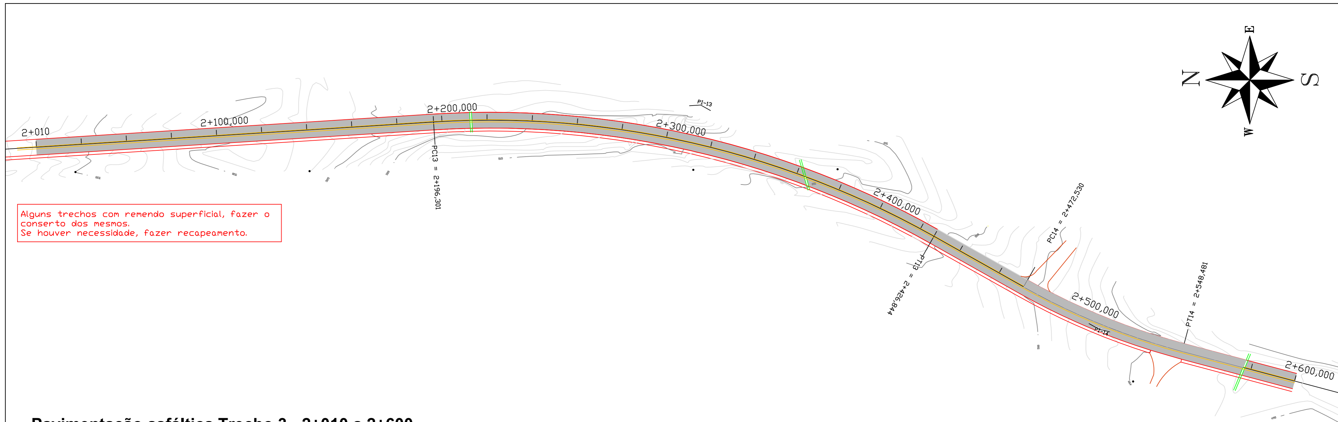
Pavimentação asfáltica Trecho 3 - 2+010 a 2+600 Escala 1/1000
