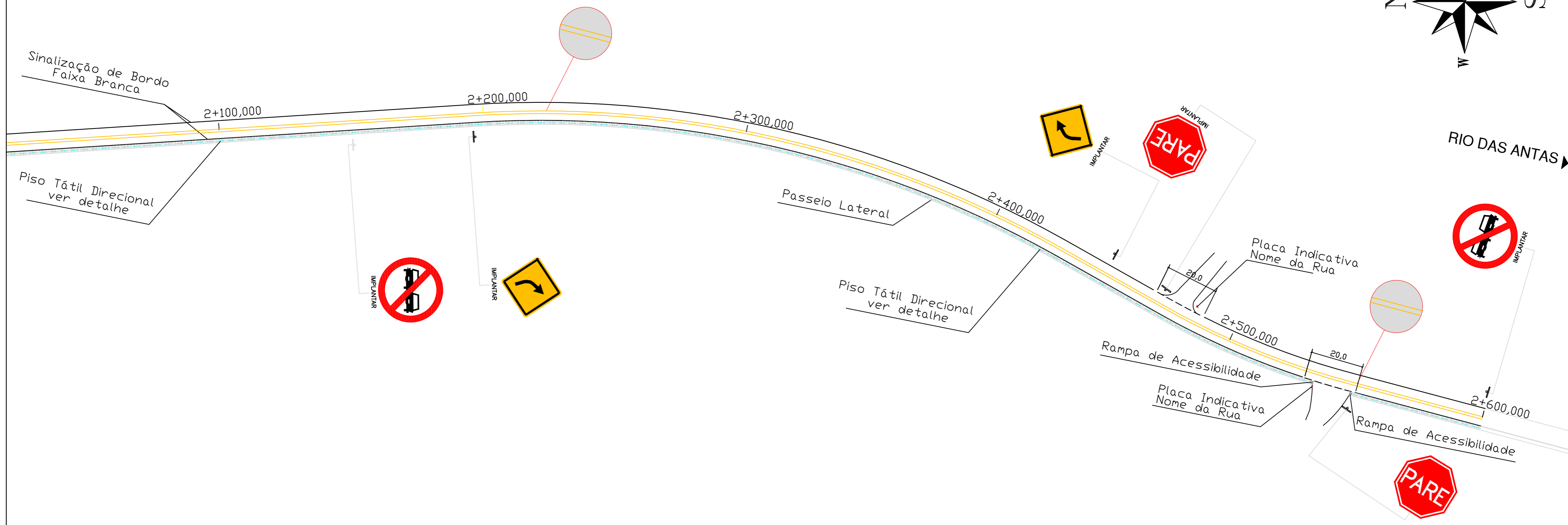
Sinalização Trecho 3 - 2+010 a 2+600 Escala 1/1000
