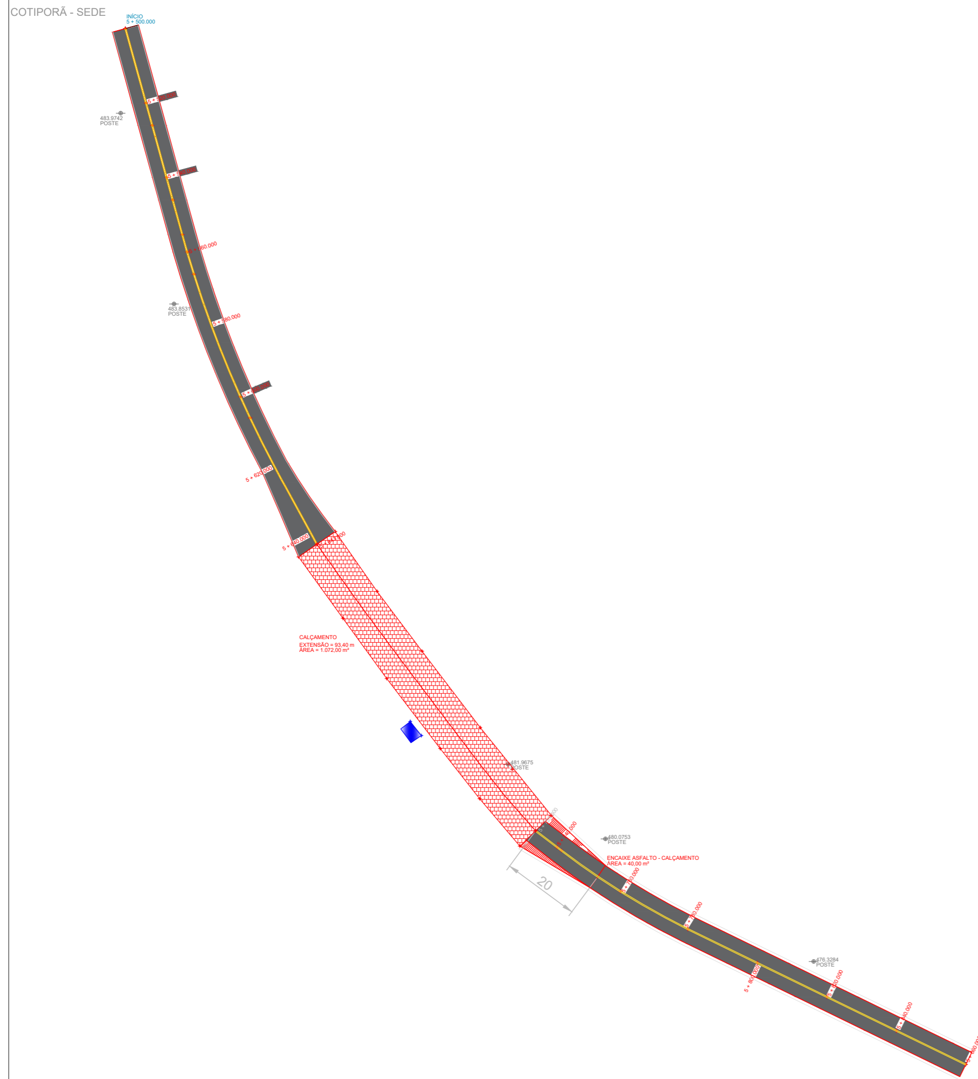
Pavimentação asfáltica Trecho 7 - 5+473 a 5+860 Escala 1/1000
