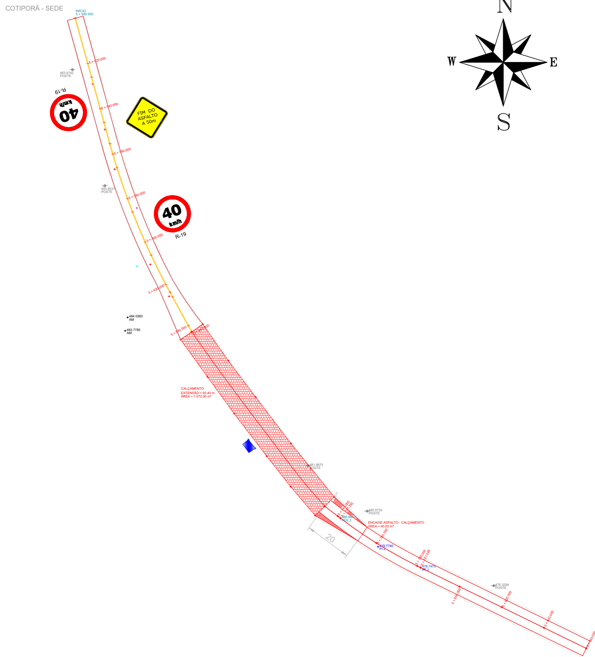
Sinalização Trecho 7 - 5+473 a 5+860 Escala 1/1000
